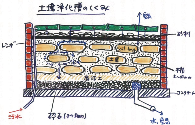
安藤家の土壌浄化槽の仕組み 図提供：安藤忠男
